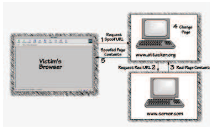
Figura 3.16: Schema riassuntivo di un attacco di tipo Web Spoofing
