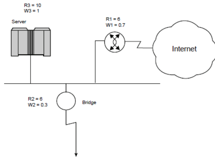
Figura 2.2: Rete d'esempio in cui per ogni componente sono stati stimati rischio e peso
