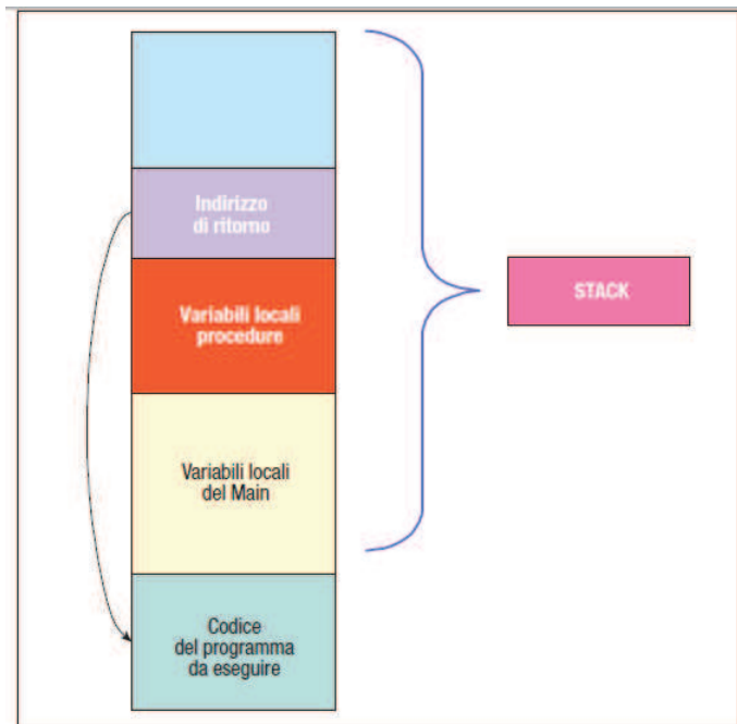
Figura 3.26: Stato dello stack in seguito alla chiamata di una procedura secondaria
