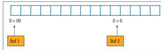
Figura 3.23: Allocazione in memoria delle variabili Buf1 e Buf2
