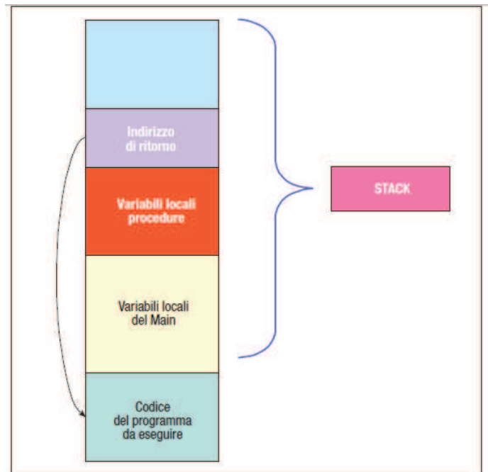
Figura 3.26: Stato dello stack in seguito alla chiamata di una procedura secondaria
