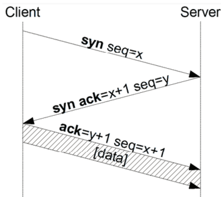
Figura 3.15: Protocollo Handshake
