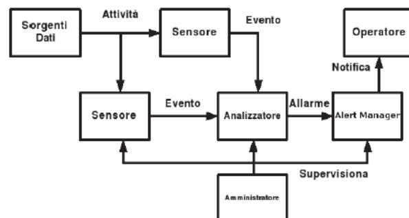
Figura 3.30: Schema funzionamento relativo agli IDS
