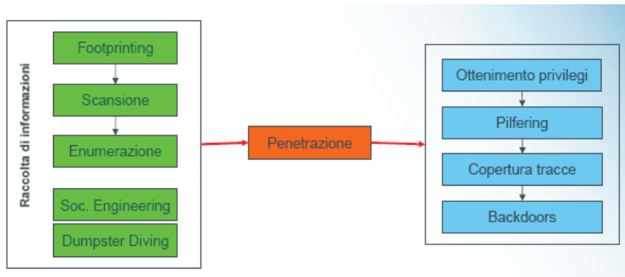
Figura 3.11: Schema relativo alle fasi di un attacco
