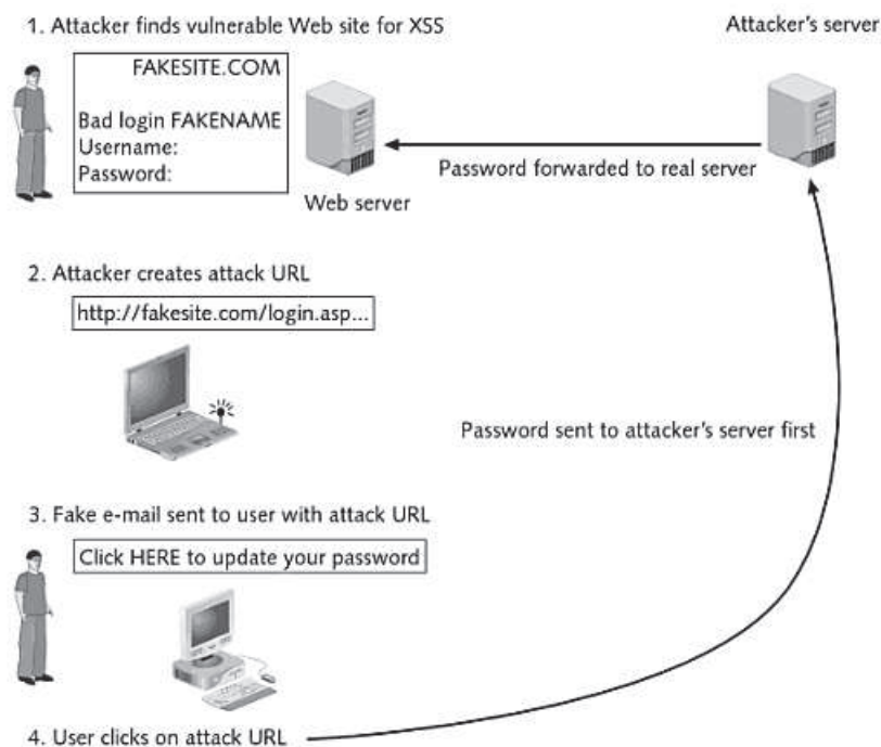
Figura 3.19: Schema riassuntivo relativo ad un attacco di tipo Cross Site Scripting
