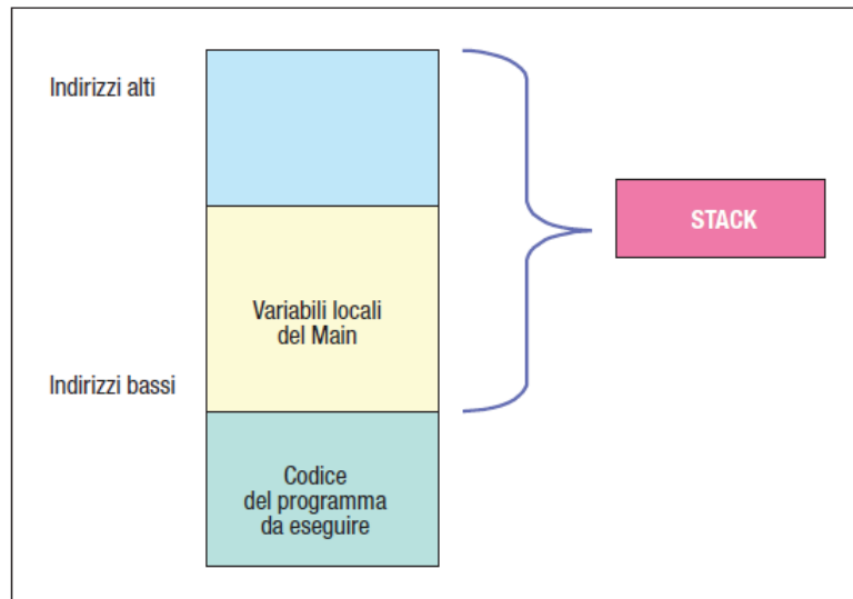
Figura 3.25: Caricamento parte dati, di un programma in esecuzione, all'interno della Memoria Centrale
