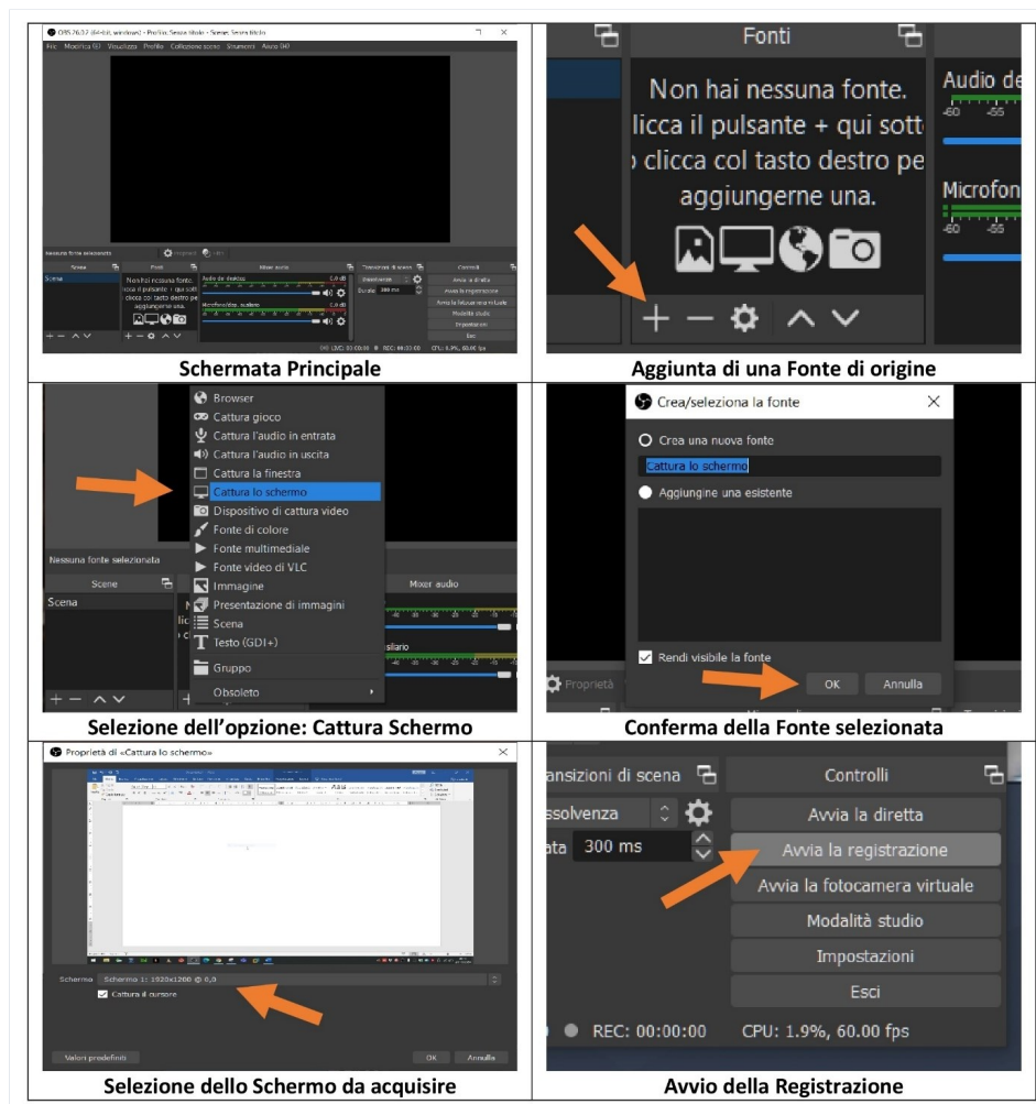
Figura 10. OBS Studio: configurazione e avvio.
