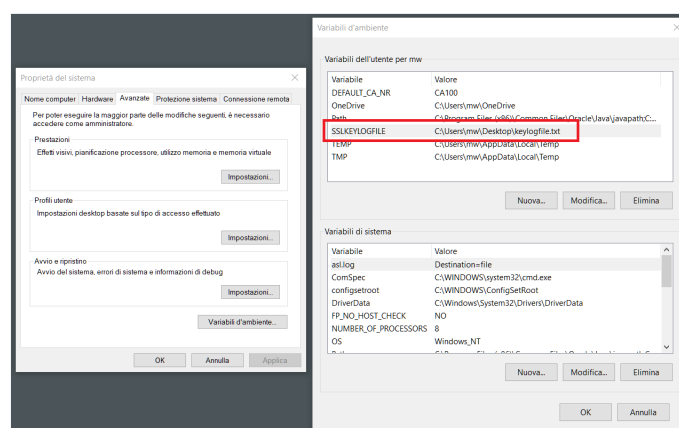
Figura 12. Impostare la variabile di ambiente SSLKEYLOGFILE.
