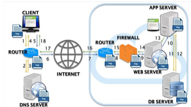
Figura 5. Schema semplificato della richiesta di una pagina web.
