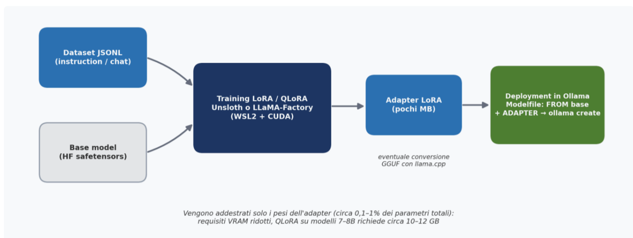
Figura 5. Workflow di fine-tuning LoRA e deployment in Ollama.
