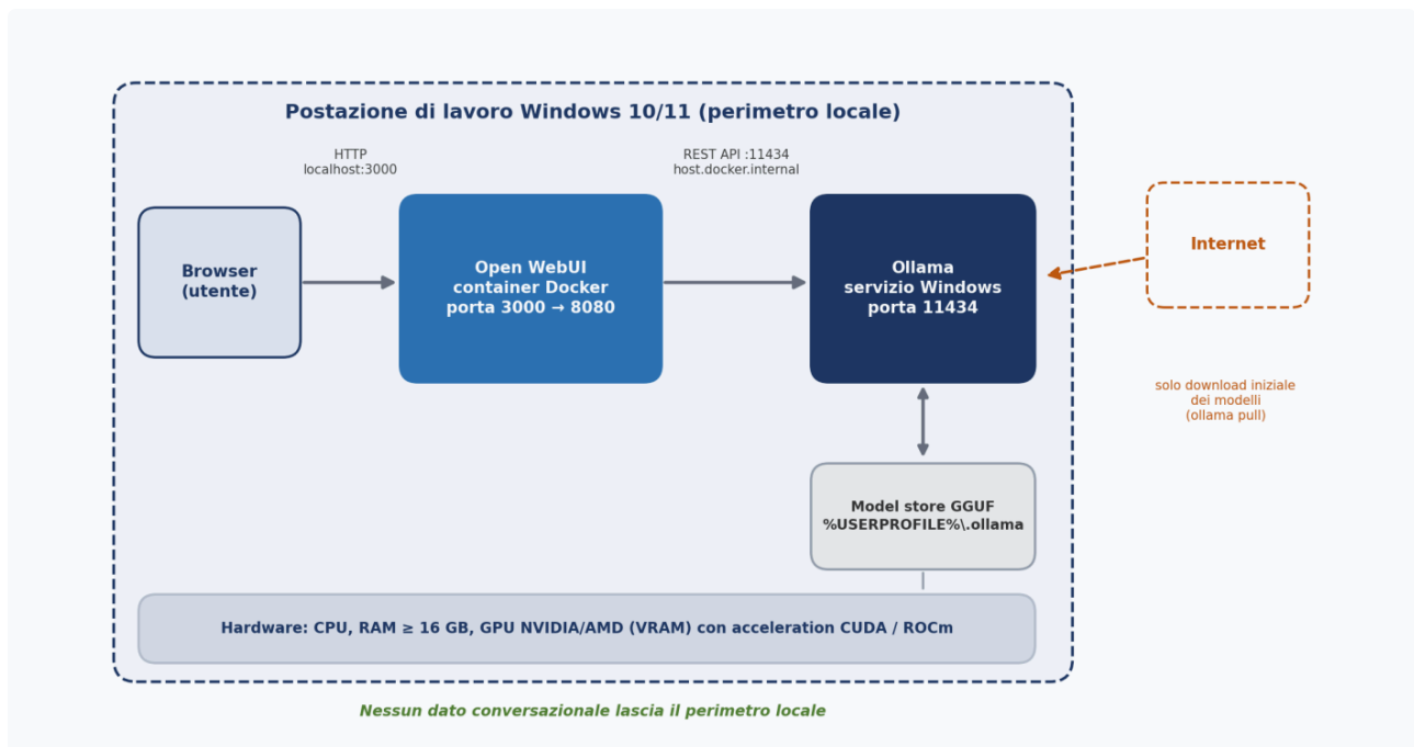
Figura 1. Architettura della soluzione: componenti, porte e perimetro locale.
