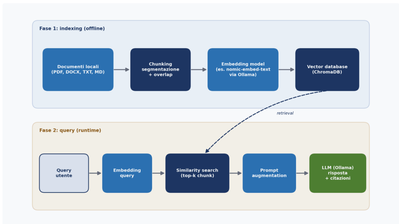
Figura 3. Pipeline RAG: fase di indexing e fase di query.
