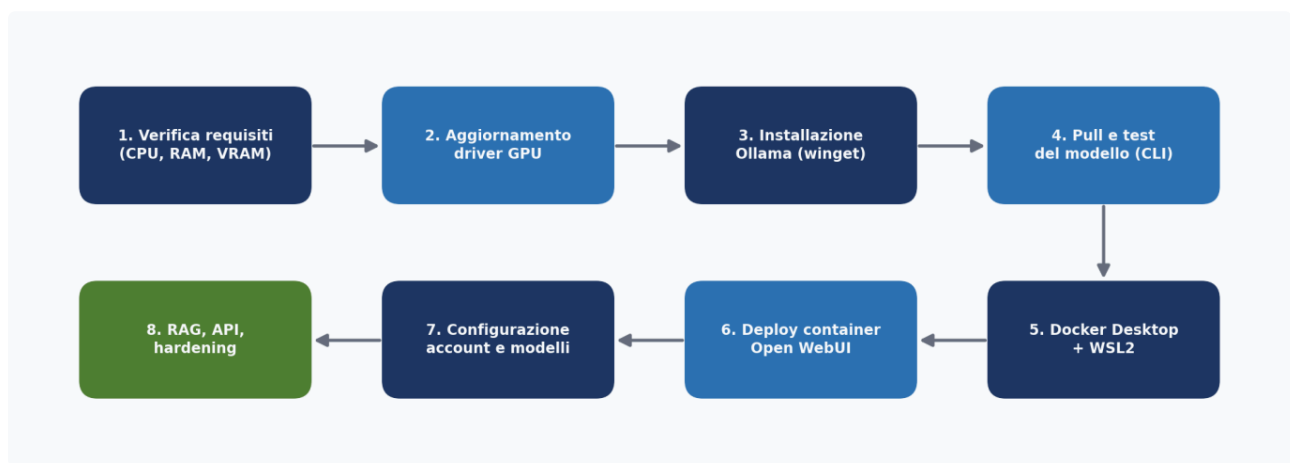
Figura 2. Flusso operativo complessivo dell'implementazione.
