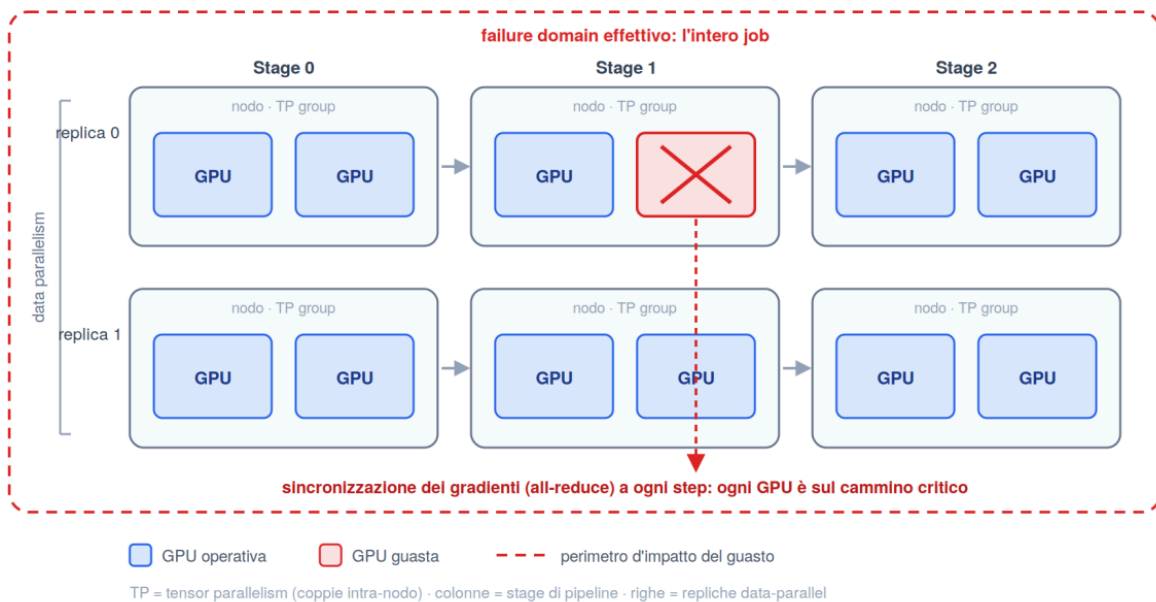
Figura 2. Composizione degli assi di parallelismo (tensor, pipeline, data) e inversione del failure domain: il guasto di un singolo acceleratore si propaga, attraverso la sincronizzazione dei gradienti, all'intero job di training.
