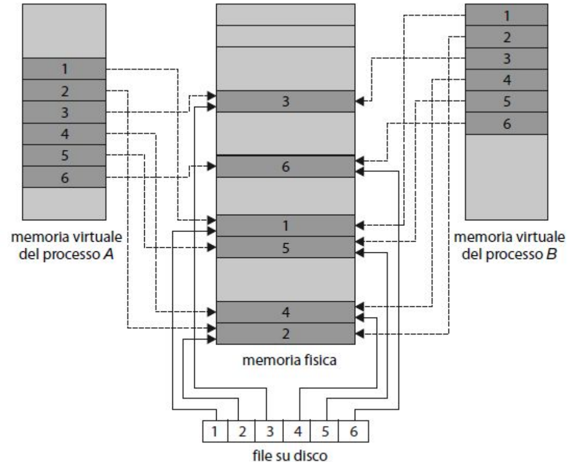
Figura 13.13 File mappati in memoria.
